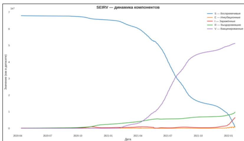
Рисунок 1 – Динамика компонентов SEIRV
