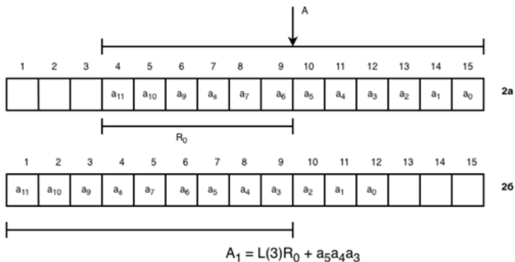
Рисунок 2 – Расположение разрядов делимого А в разрядности регистра РгА
