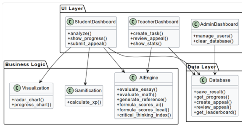
Рисунок 2 – Диаграмма компонент
