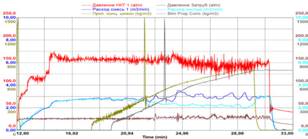
Рисунок 7 — График ГРП
