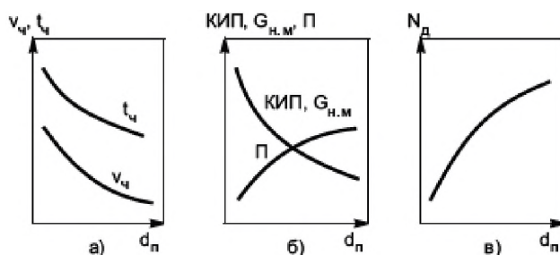
Рис. 1 – Зависимость параметров плазменного напыления: скорости V_n и температуры t_n частиц (а), КИП, производительности и пористости покрытия \Pi (б), мощности дуги N_d (в) от диаметра d_n частиц порошка
